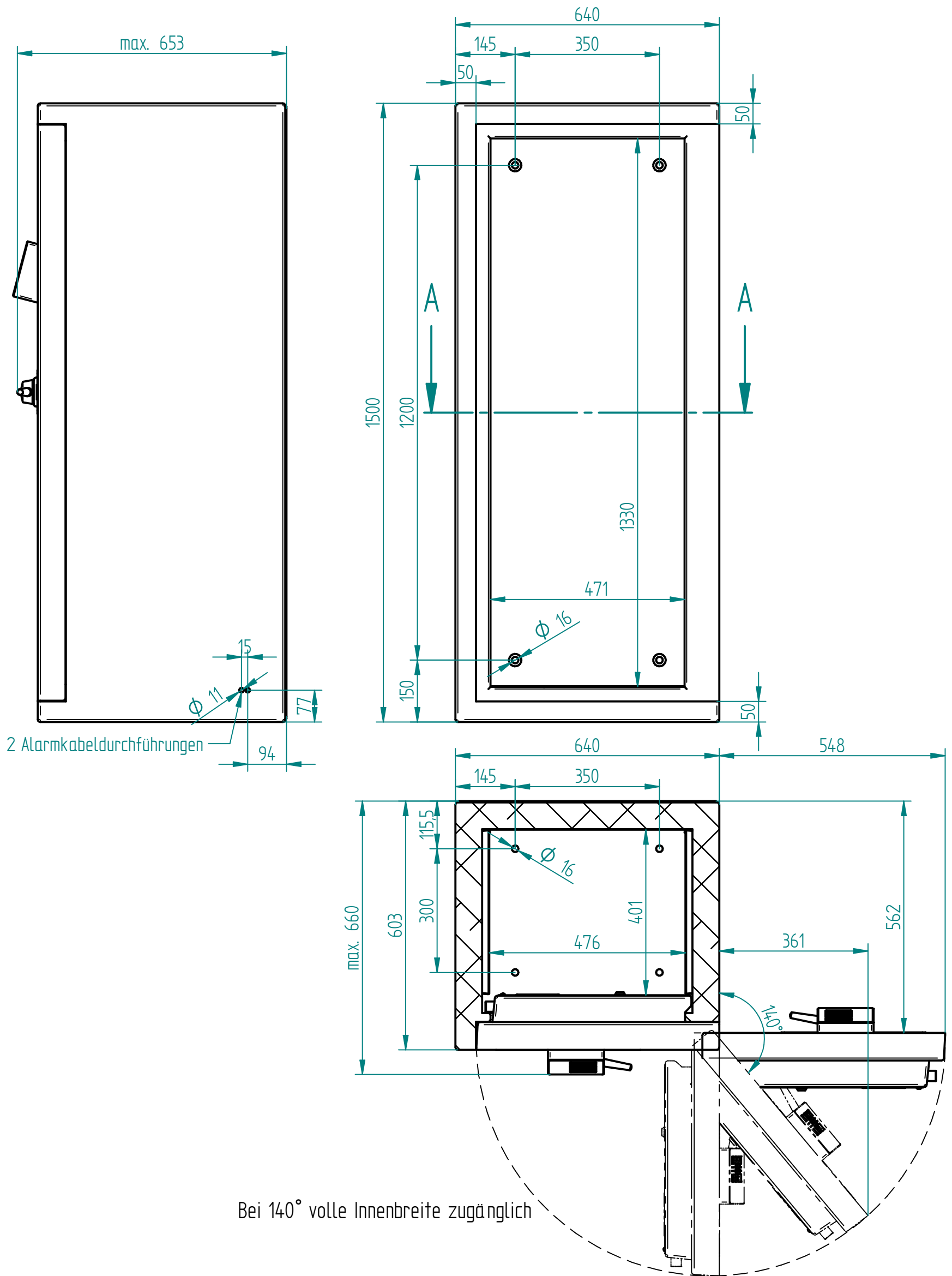
Schnitt A-A
