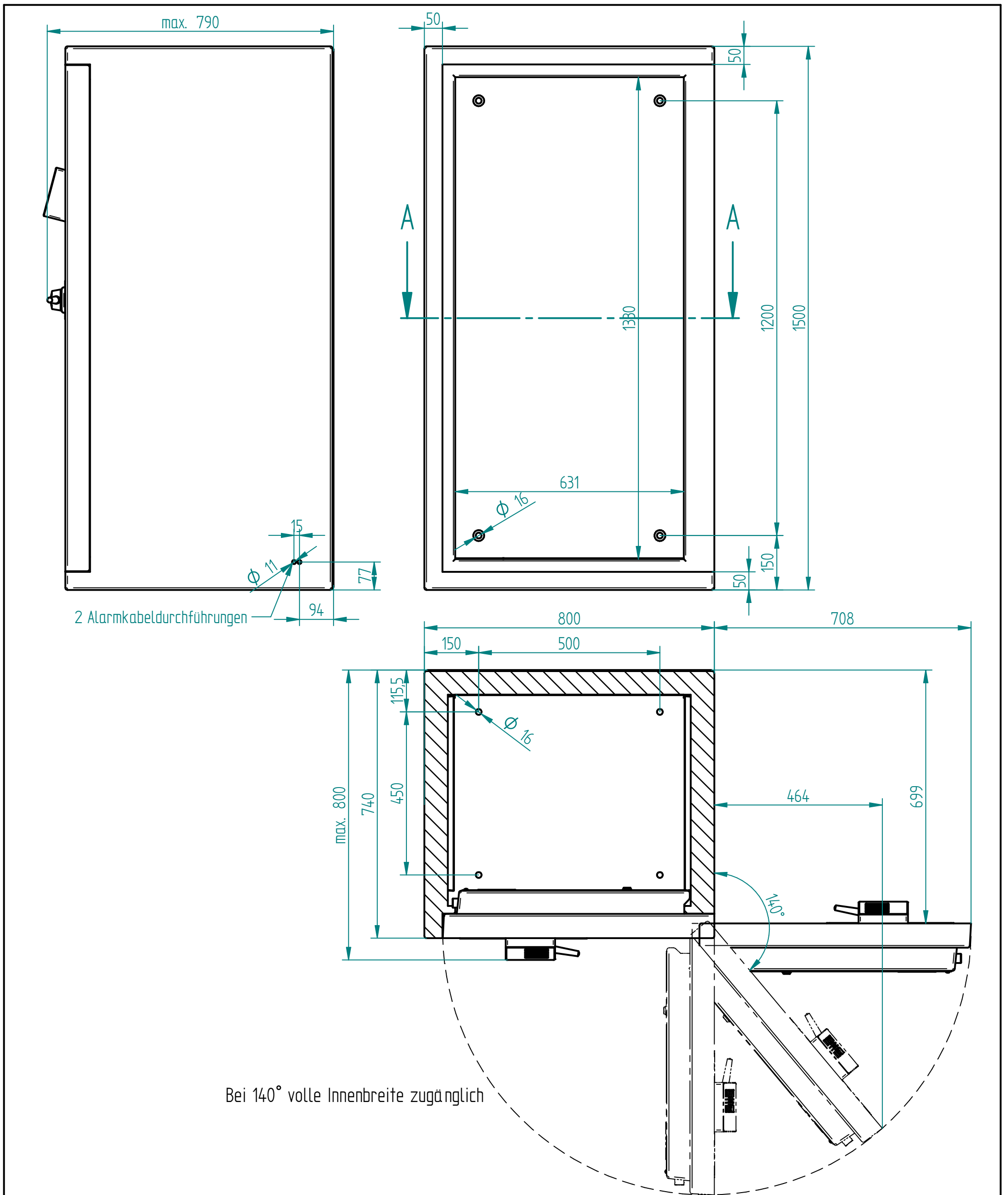
Schnitt A-A
